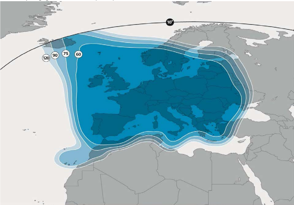
Bild: Empfangsgebiet ASTRA 1N (SDTV)
